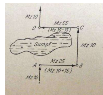
Umgehen im rechten Winkel
