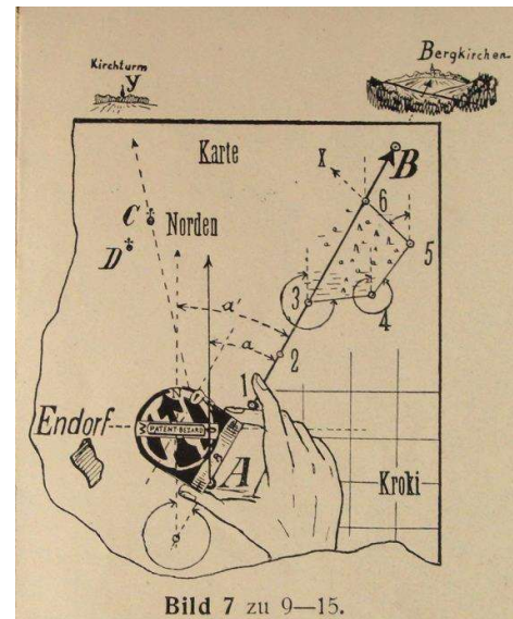
Anlegen des Bézard Kompasses an die Richtungslinie
