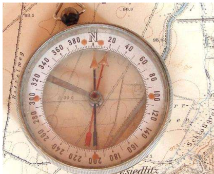
Kartenkompass S-L aus den 1930er Jahren
