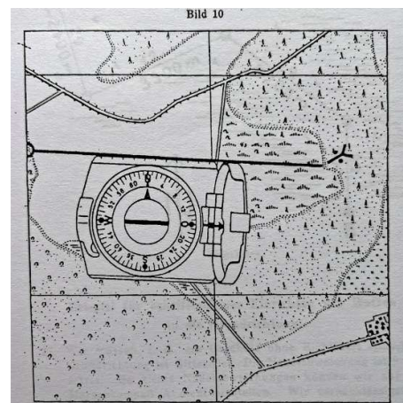
Übertragen einer Richtung in die Karte
