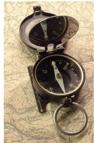
Einrichten der Karte Modell mit Nadelarretierung
