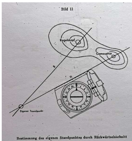
Rückwärtseinschneiden
