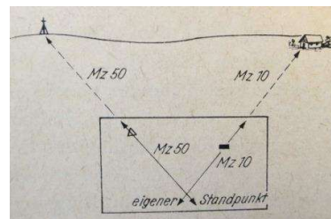
Rückwärtseinschneiden
