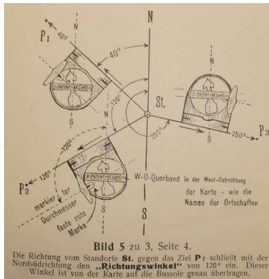
Ermitteln von Richtungswinkel zum Ziel
