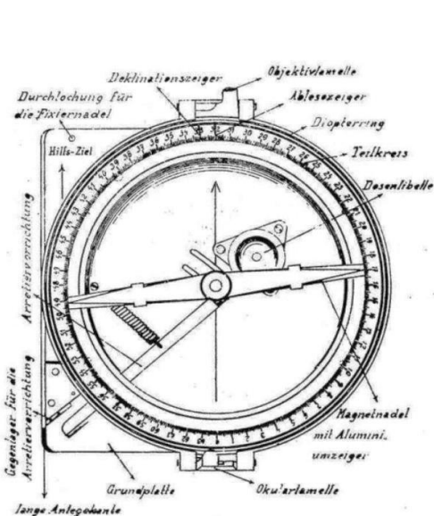
Richtbussole M 15
